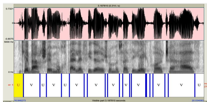
شکل ۱: نمونه‌ای از نحوه جداسازی مناطق واکه‌دار و بی‌واک سیگنال‌های آوایی
